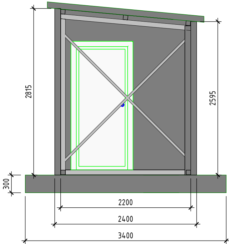
Разрез 2-2
