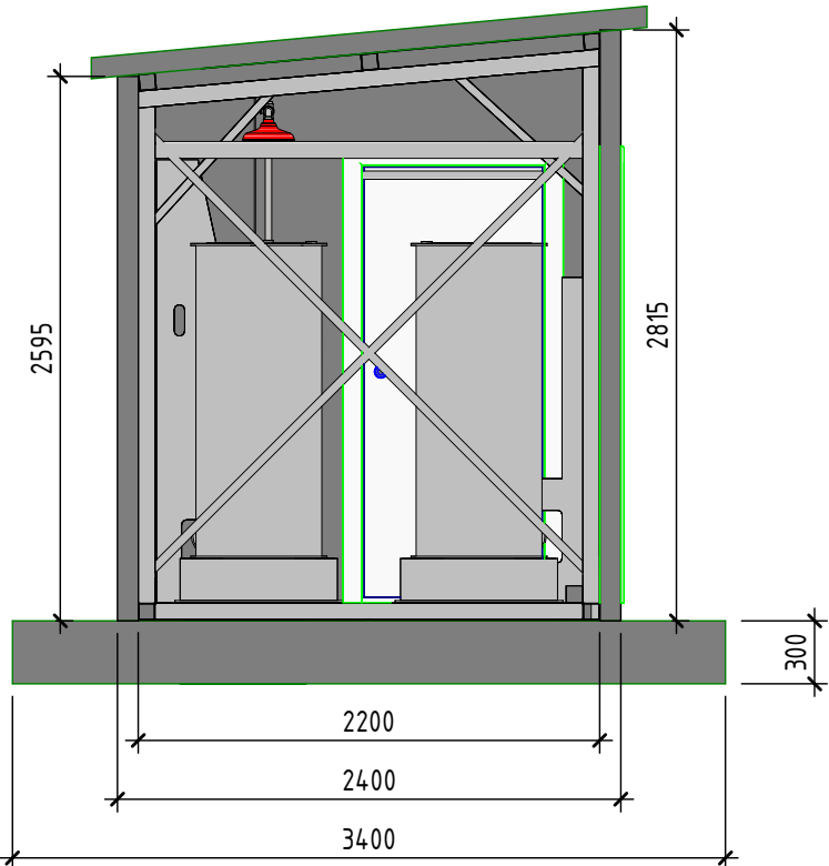
Разрез 3-3
