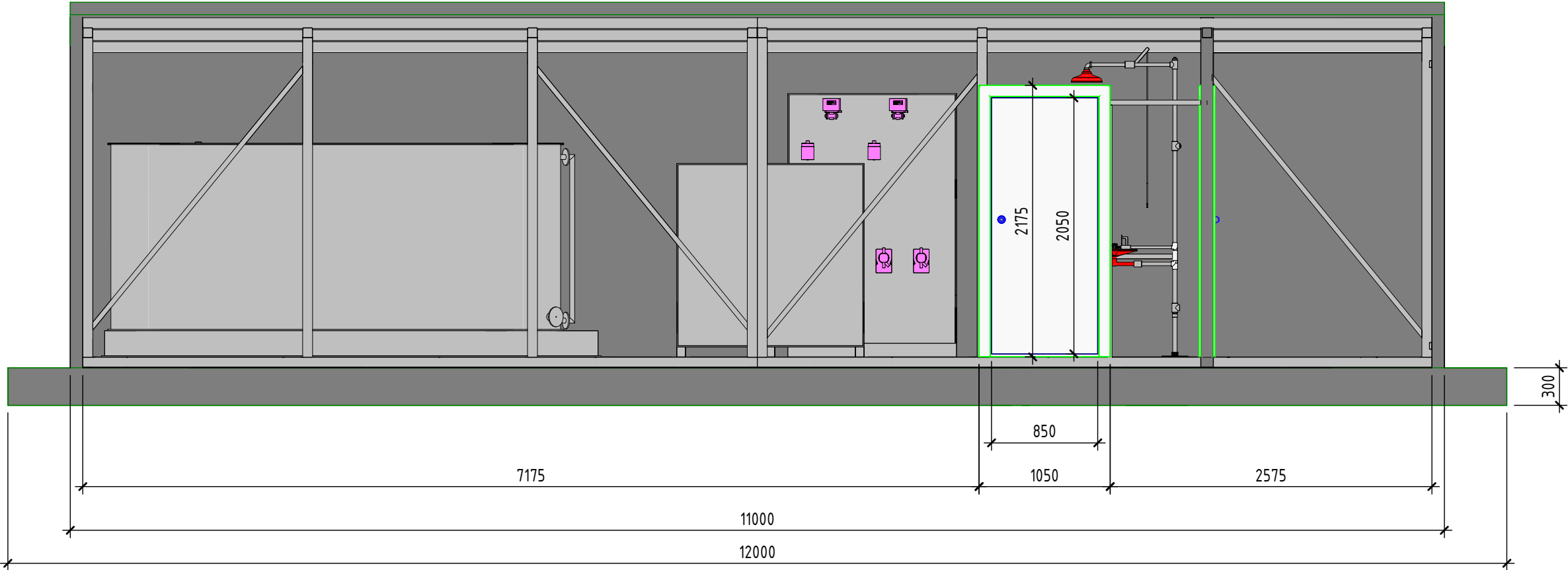
Разрез 1-1
